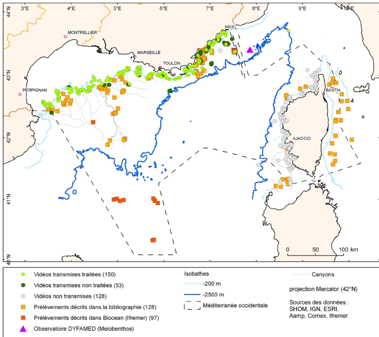
Figure 1 : Localisation géographique des données existantes sur substrat meuble en Méditerranée occidentale (golfe du Lion, mer Ligure) dans les zones bathyales et abyssales (Sources : SHOM, IGN, ESRI, AAMP, Comex, Ifremer, 2012).
