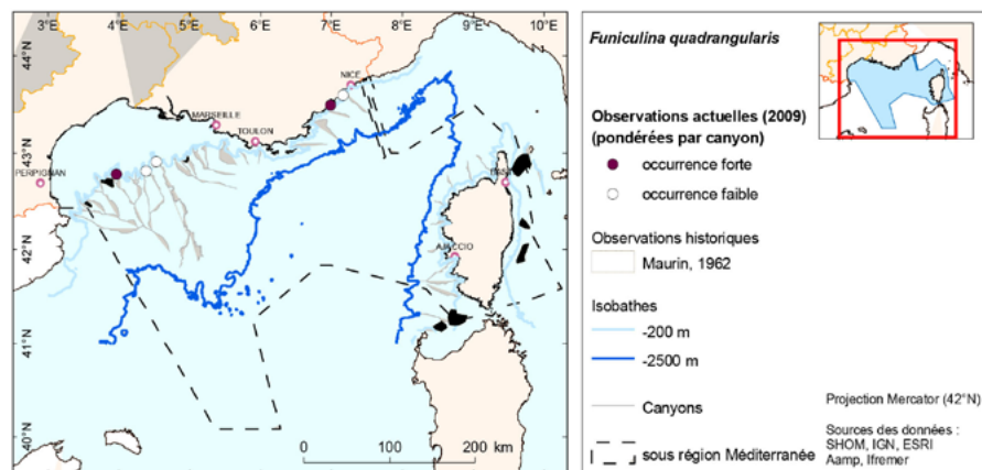
Figure 3 : Carte de localisation des vases molles à Funiculina quadrangularis observées pendant la campagne MEDSEACAN 2009 et dans les données historiques en Méditerranée occidentale. Elles ont probablement été observées pendant la campagne CORSEACAN 2010, mais les vidéos n'ont pas pu être visionnées dans le cadre de l'état initial de la DCSMM (Sources : SHOM, IGN, ESRI, AAMP, Ifremer, 2012).
