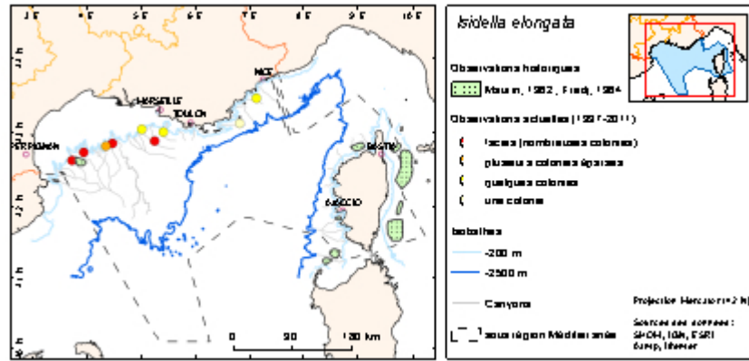
Figure 2 : Carte de localisation des Isidella elongata observées pendant les campagnes MEDSEACAN 2009, Cylice 1997, ESSNAUT2008, ESSROV2010, 2011 et dans les données historiques en Méditerranée occidentale. Elles ont probablement été observées pendant la campagne CORSEACAN 2010, mais les vidéos n'ont pas pu être visionnées dans le cadre de l'état initial de la DCSMM (Sources : SHOM, IGN, ESRI, AAMP, Ifremer, 2012).
